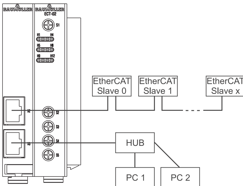
Abbildung 14: Beispiel einer Konfiguration Modul Ethernet mit EtherCAT-Master
