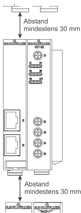
Abbildung 5: Einbauraum b maXX System
