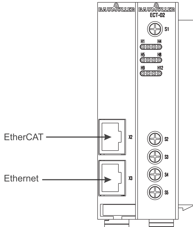
Abbildung 12: Anschlussbild Ethernet mit EtherCAT-Master für b maXX controller PLC
