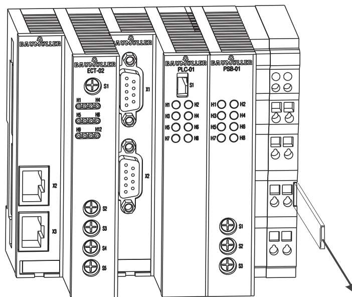
Abbildung 9: Ethernet mit EtherCAT-Master, b maXX controller PLC, Netzteil
