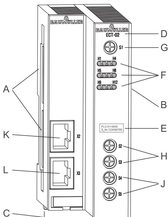
Abbildung 1: Modul Ethernet mit EtherCAT-Master
