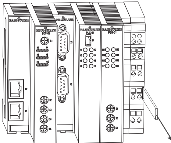
Abbildung 18: Ethernet mit EtherCAT-Master, b maXX controller PLC, Netzteil
