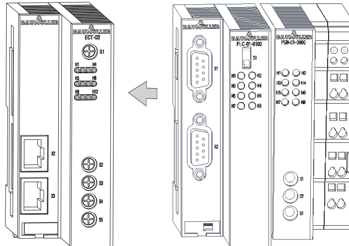
Abbildung 7: Ethernet mit EtherCAT-Master + b maXX controller PLC und Netzteil
