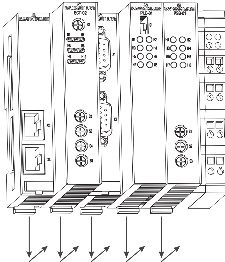
Abbildung 8: Ethernet mit EtherCAT-Master, b maXX controller PLC und Netzteil
