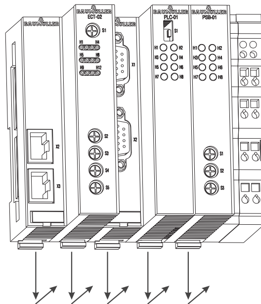
Abbildung 17: Ethernet mit EtherCAT-Master, b maXX controller PLC und Netzteil
