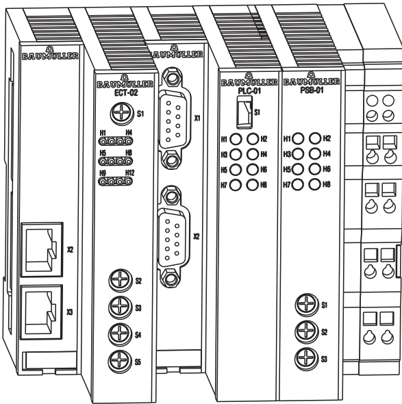
Abbildung 2: Ethernet mit EtherCAT-Master + b maXX controller PLC und Netzteil
