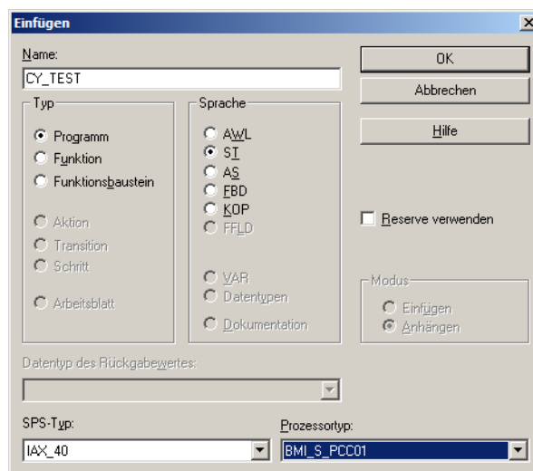
Abbildung 40: Anlegen einer neuen POE mit Spezialisierung auf Prozessortyp
