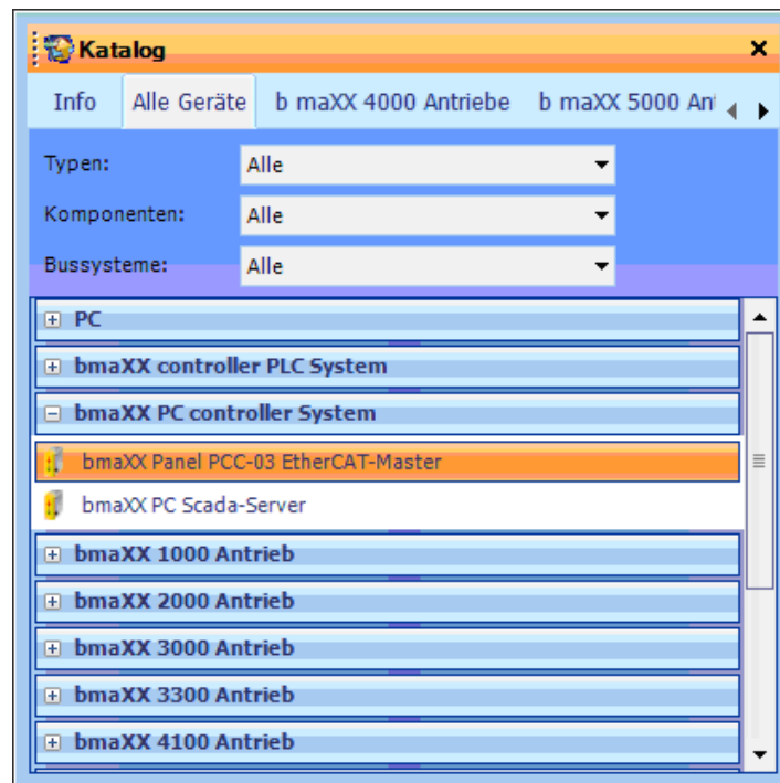
Abbildung 16: ProMaster-Katalog mit Einträgen für PCC-03
