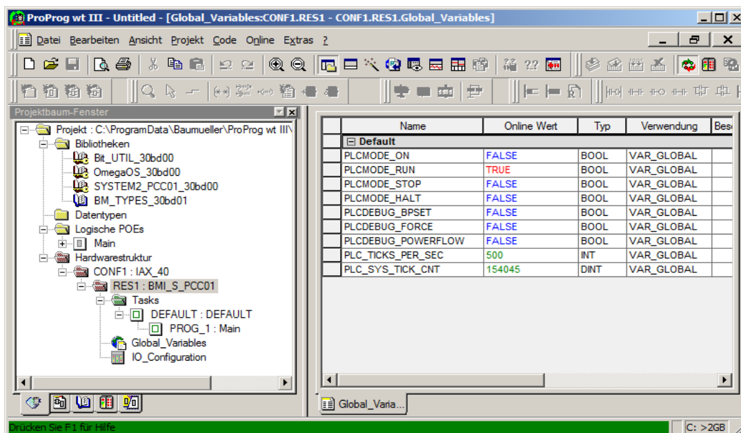
Abbildung 26: Das Arbeitsblatt „Global_Variables“ im Debug-Modus
