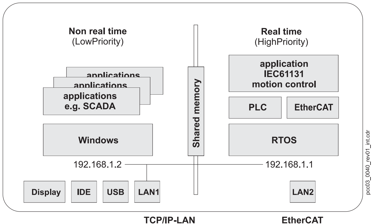
Abbildung 1: Teilung Echtzeit/Nicht-Echtzeit
