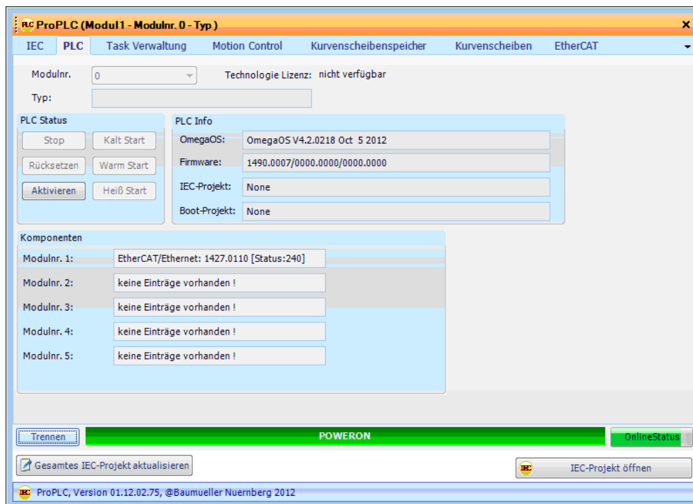
Abbildung 19: ProMaster verbunden mit b maXX-PLC des PCC-03
