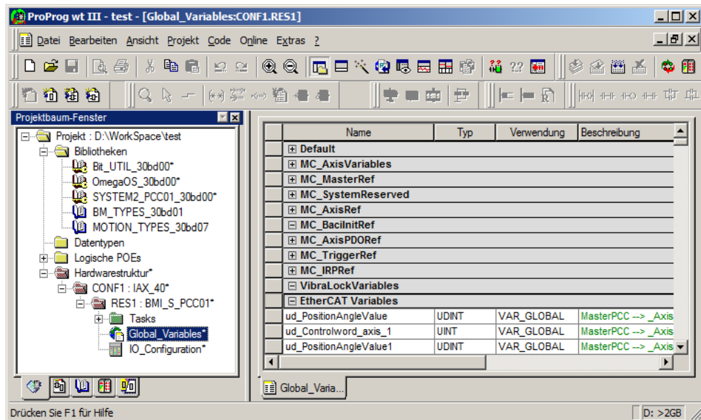
Abbildung 29: Nach dem Export
