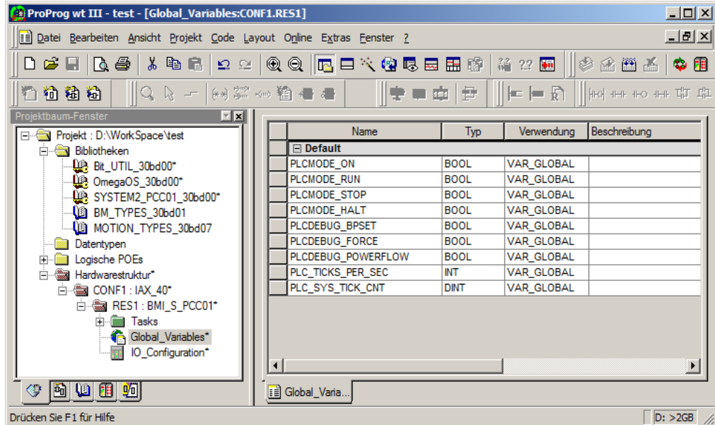
Abbildung 28: Vor dem Export
