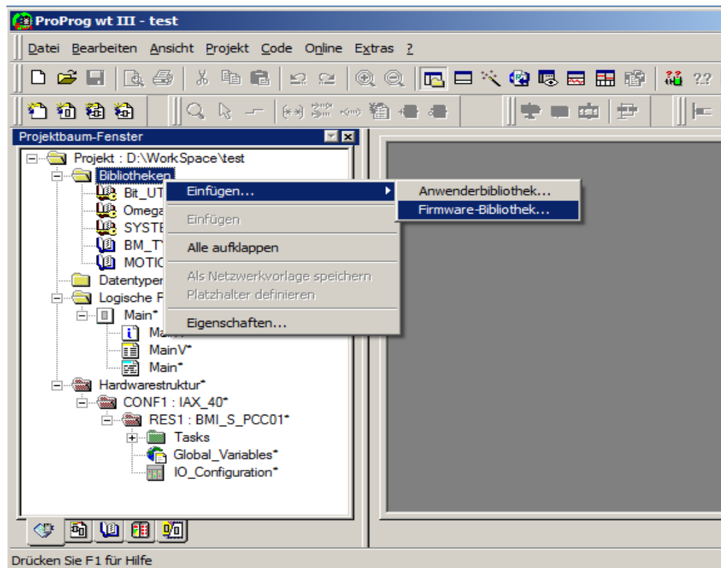
Abbildung 37: Einbinden von Firmware-Bibliotheken
