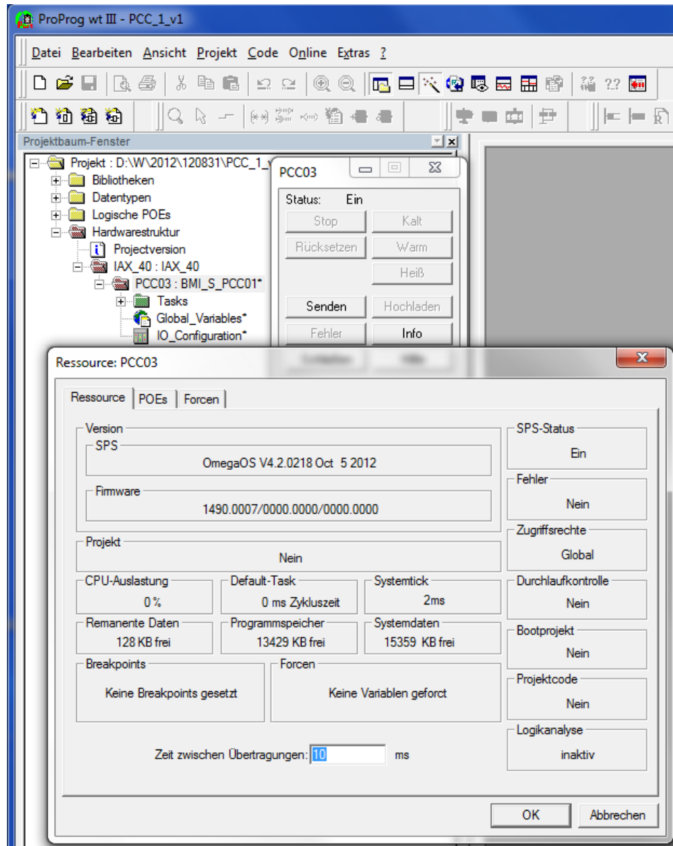
Abbildung 6: Erster Zugriff mit ProProg wt III auf die b maXX-PLC des PCC-03
