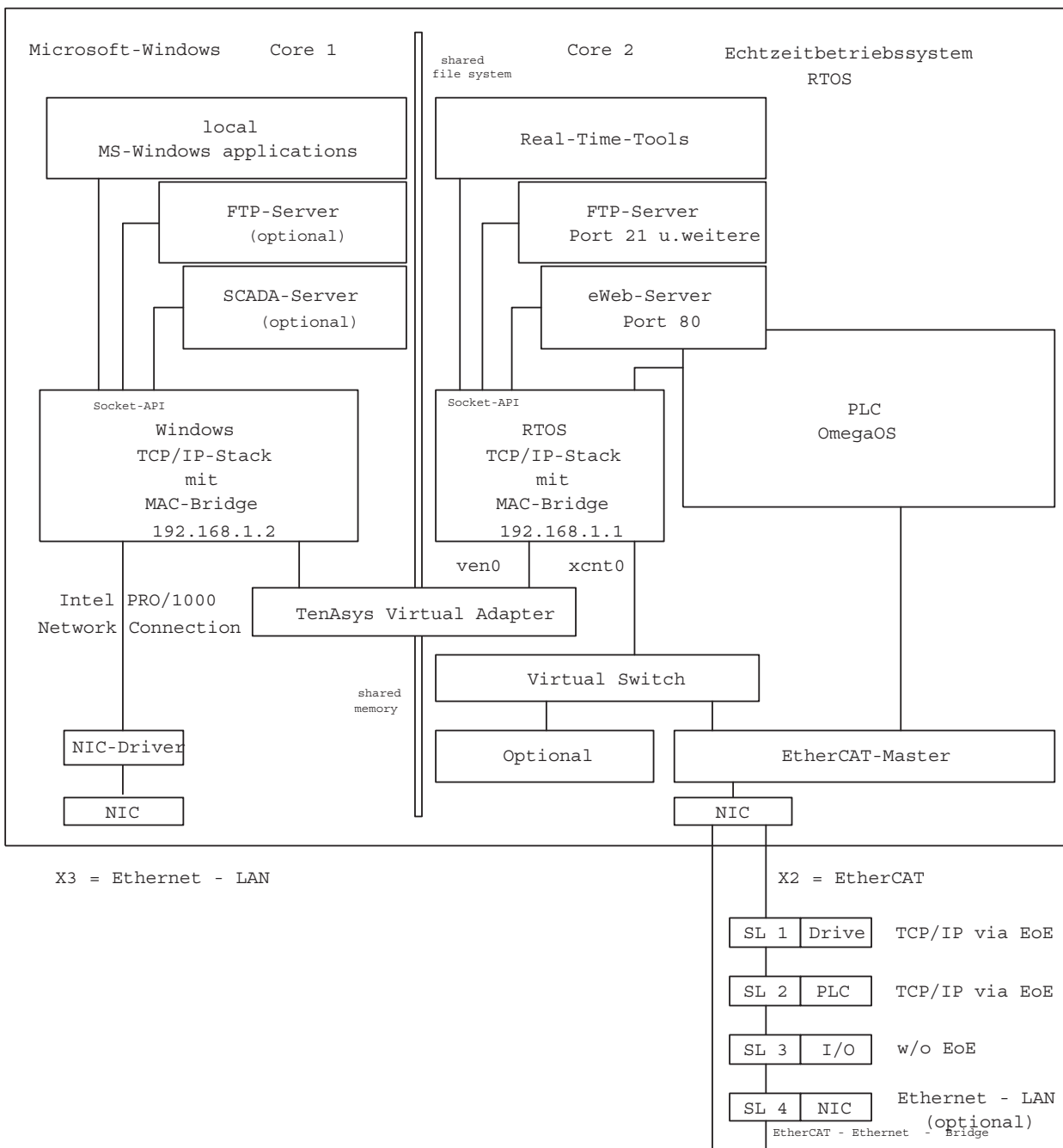
Abbildung 8: TCP/IP-Kommunikations-Schema des PCC-03.
