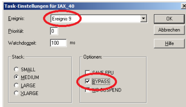
Abbildung 33: Eigenschaften der neuen Task 2
